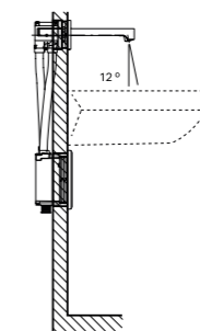
↑ RUBINETTERIA GEBERIT BRENTA Montaggio a parete
