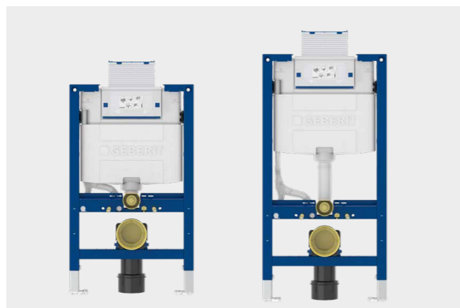
↑ Modulo Geberit Duofix Omega per WC, 82 cm e 98 cm, con cassetta di risciacquo Omega 12 cm, permette di azionare il risciacquo dall'alto o frontale. La soluzione ideale per realizzare un bagno in locali mansardati o sotto la mensola di una finestra.
