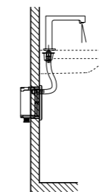
↑ RUBINETTERIA GEBERIT BRENTA Montaggio a pianale
